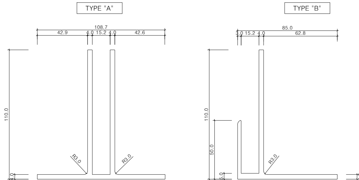
하부고정철물(W15) 상세도
