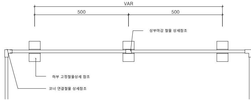
멀티엣지(W15) H200 평면도
