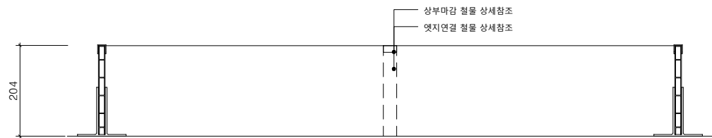
멀티엣지(W15) H200 정면도
