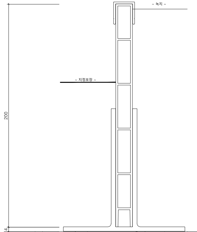
멀티엣지(W15) H200단면도
