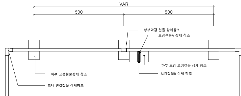
멀티엣지(W15) H250 평면도
