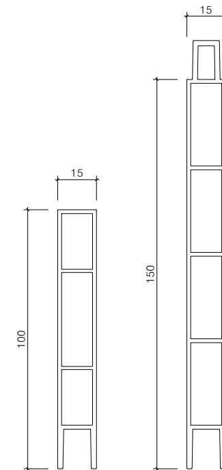
멀티엣지(W15) 알루미늄구조도(H100,150)
