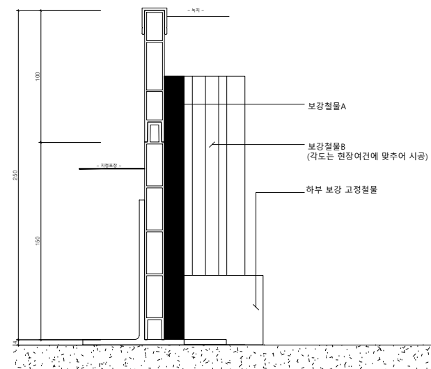
멀티엣지(W15) H250단면도
