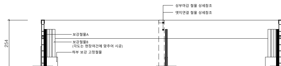
멀티엣지(W15) H250 정면도
