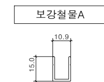
멀티엣지(W15) 알루미늄구조도(H150) SCALE : A1=1/1, A3=1/2
