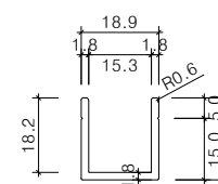
연결철물(W15) 상세도 SCALE : NONE
