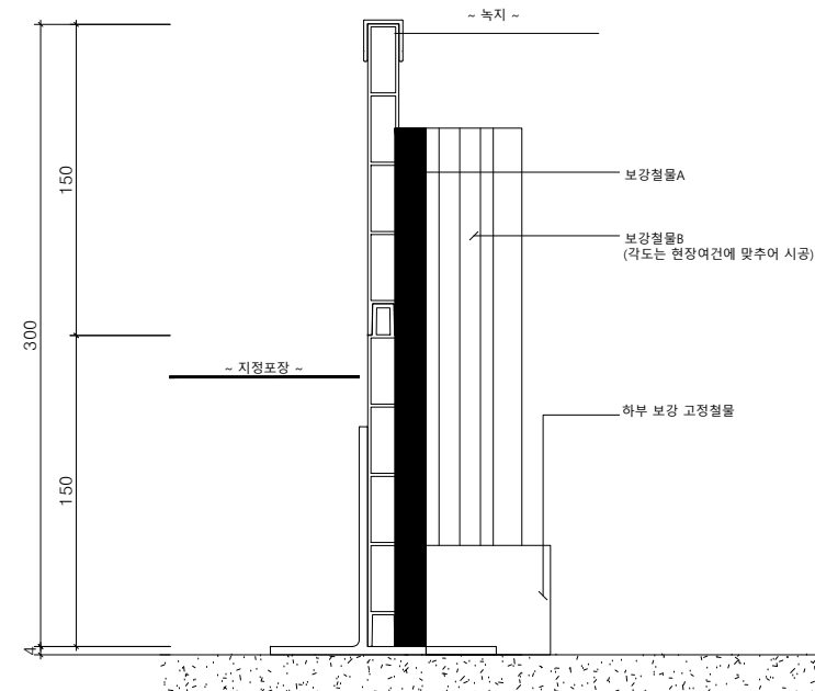
멀티엣지(W15) H300단면도 SCALE : A1=1/2, A3=1/4
