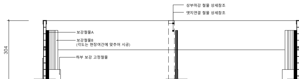
멀티엣지(W15) H300 정면도
