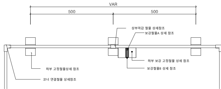
멀티엣지(W15) H300 평면도 SCALE : A1=1/6, A3=1/12
