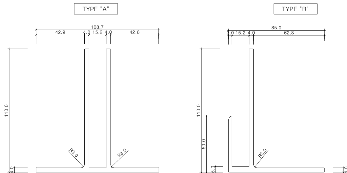
하부고정철물(W15) 상세도
