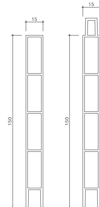
멀티엣지(W15) 알루미늄구조도(H150) SCALE : A1=1/1, A3=1/2
