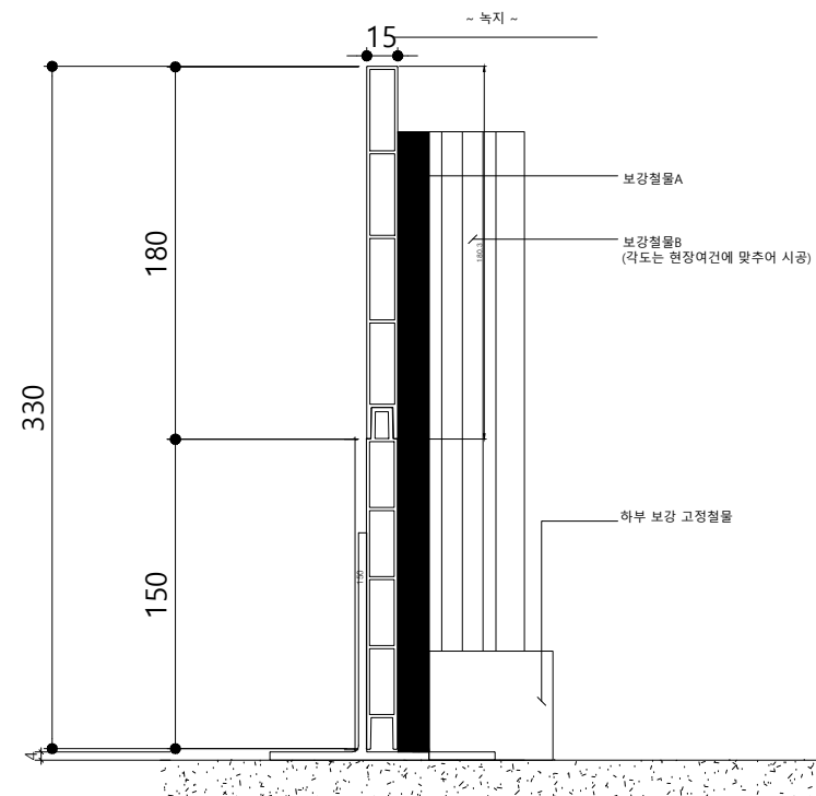
멀티엣지(W15) H350단면도
