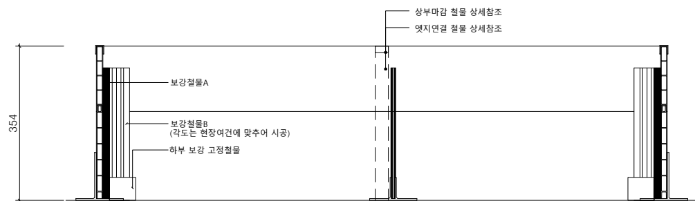
멀티엣지(W15) H350 정면도
