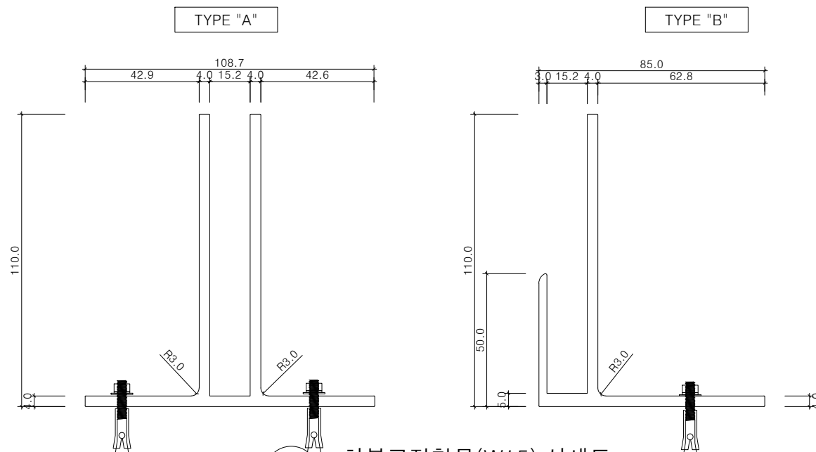
하부고정철물(W15) 상세도
