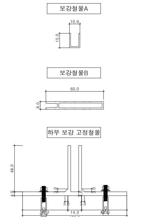
보강철물 상세도
