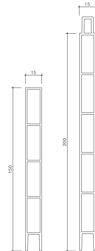
멀티엣지(W15) 알루미늄구조도(H150,200)
