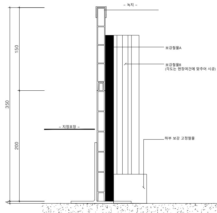
멀티엣지(W15) H350단면도
