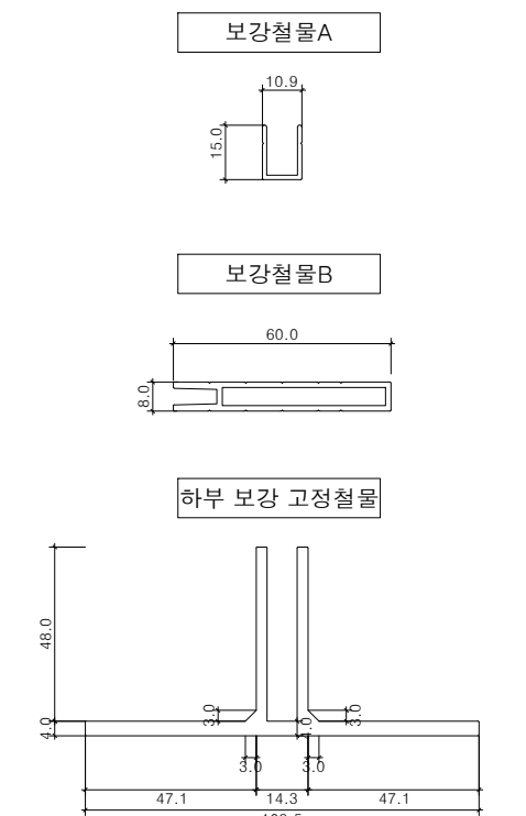
보강철물 상세도
