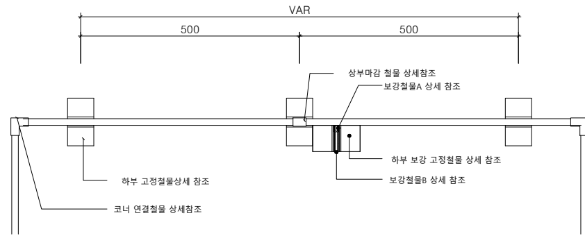
멀티엣지(W15) H350 평면도
