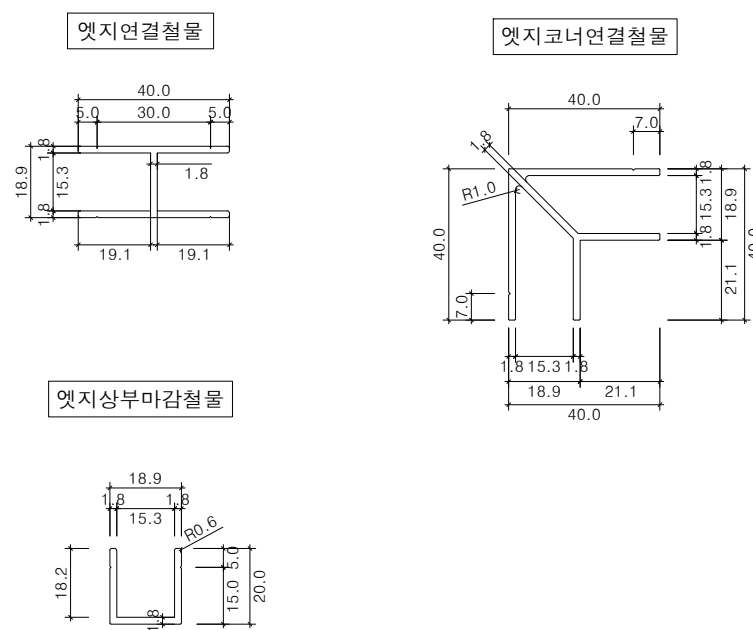
연결철물(W15) 상세도
