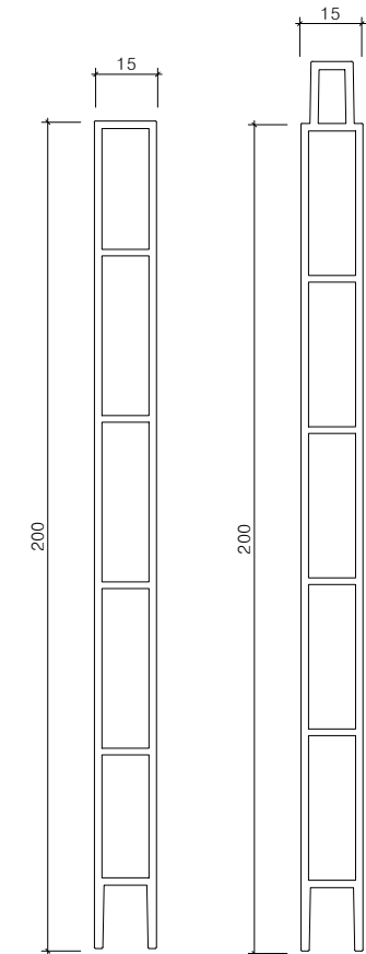
멀티엣지(W15) 알루미늄구조도(H200)
