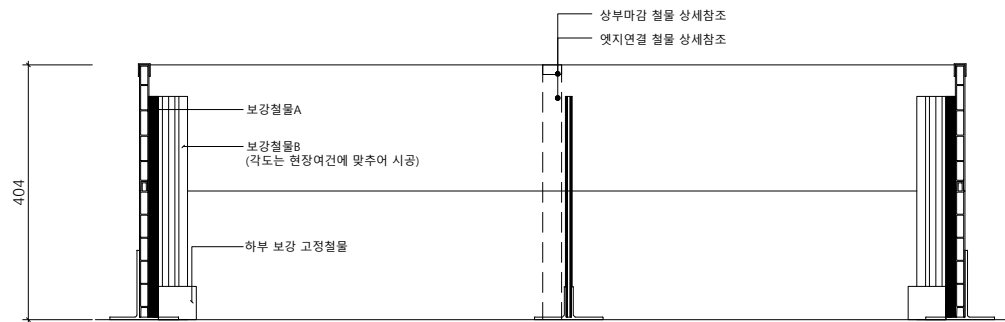
멀티엣지(W15) H400 정면도
