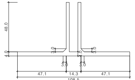
보강철물 상세도
