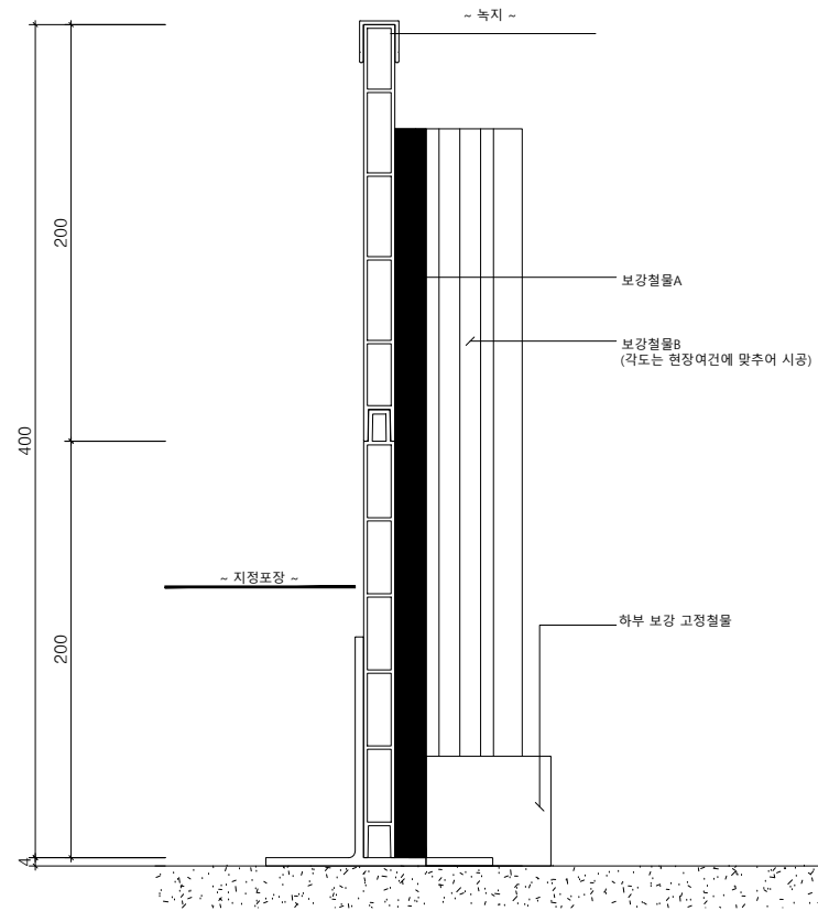
멀티엣지(W15) H400단면도
