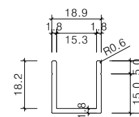
엣지상부마감철물
