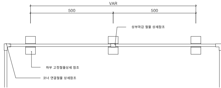
멀티엣지(W15) H400 평면도
