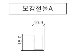
보강철물A
