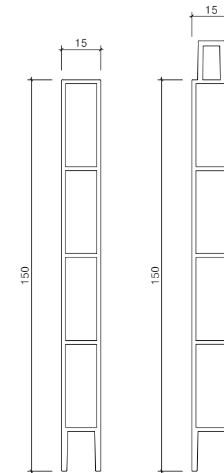
멀티엣지(W15) 알루미늄구조도(H150)
