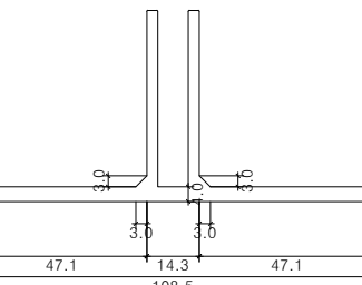
보강철물 상세도
