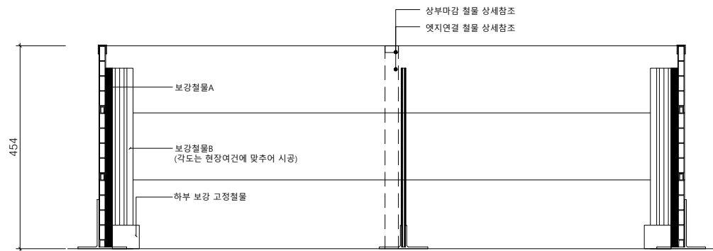
멀티엣지(W15) H450 정면도
