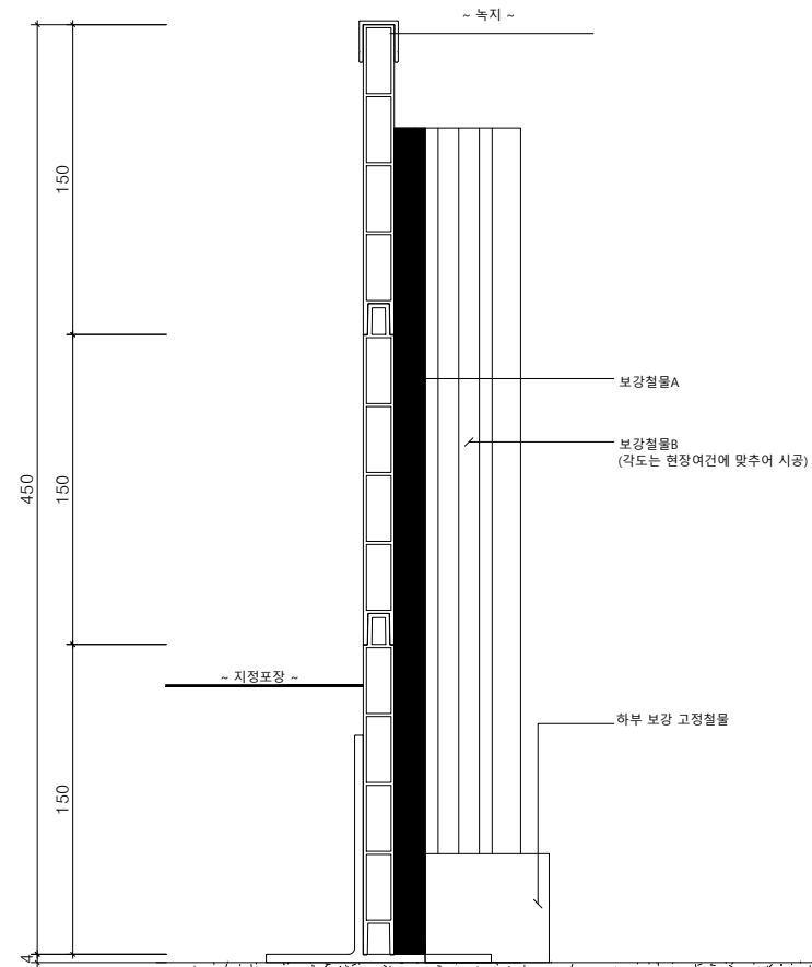
멀티엣지(W15) H450단면도
