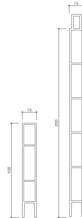
멀티엣지(W15) 알루미늄구조도(H100,200)
