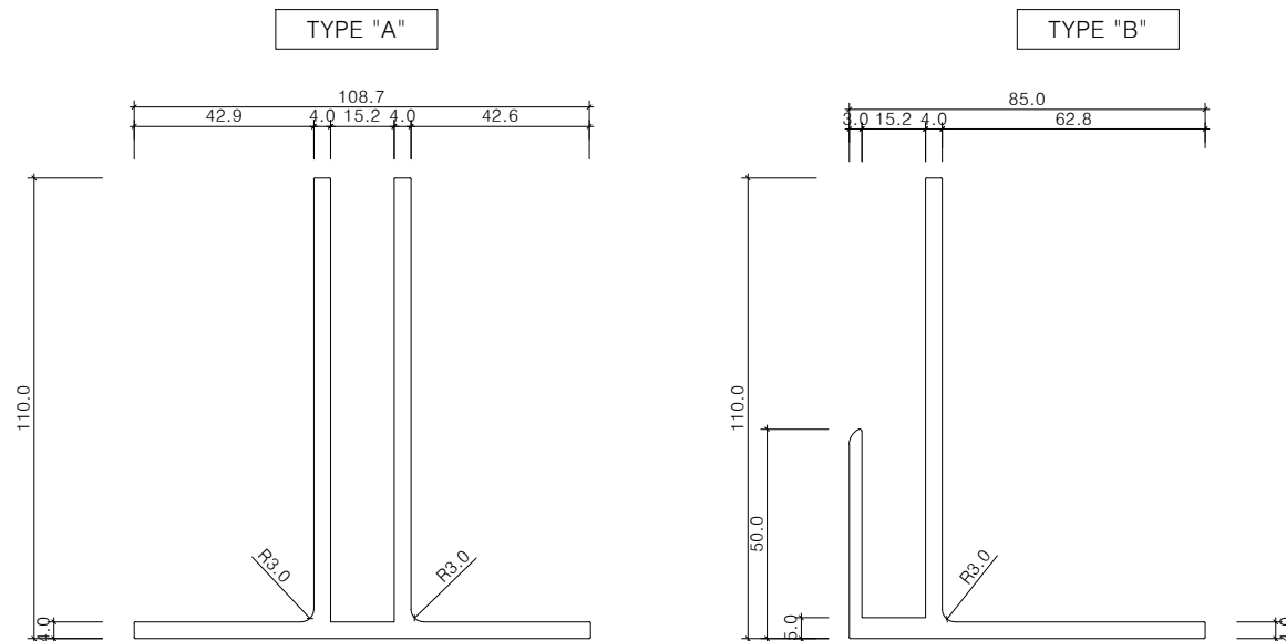
하부고정철물(W15) 상세도
