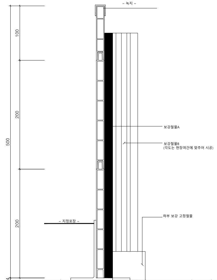
멀티엣지(W15) H500단면도
