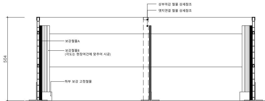
멀티엣지(W15) H500 정면도
