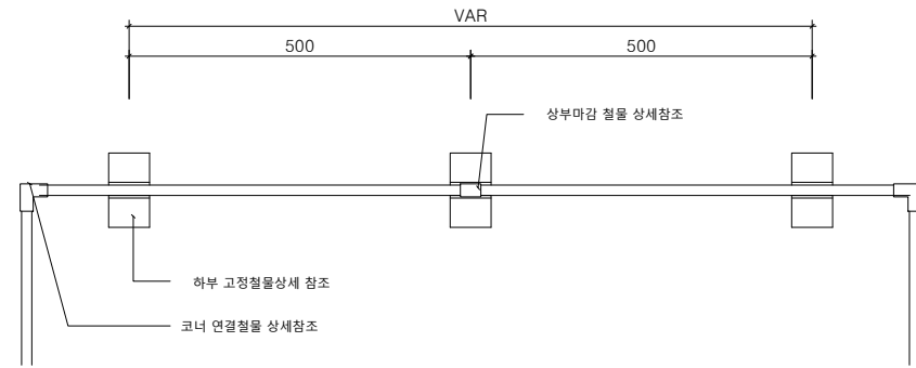
멀티엣지(W15) H500 평면도
