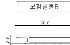
하부 보강 고정철물
