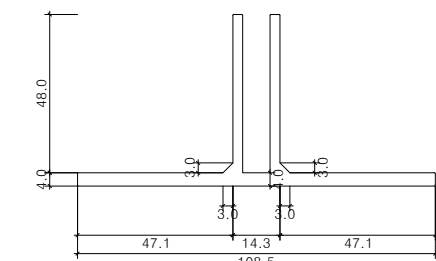
보강철물 상세도
