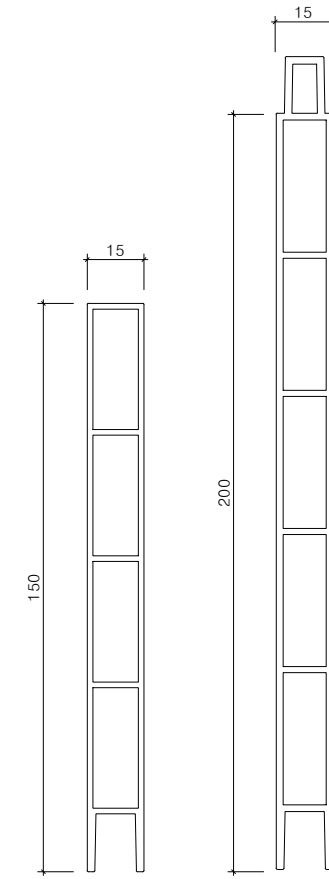
멀티엣지(W15) 알루미늄구조도(H150,200) SCALE : A1=1/1, A3=1/2
