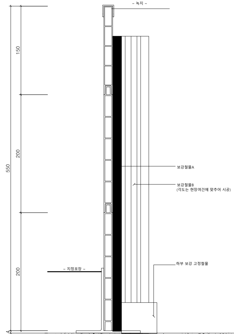
멀티엣지(W15) H550단면도 SCALE : A1=1/2, A3=1/4
