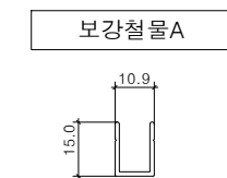
멀티엣지(W15) 알루미늄구조도(H150,200) SCALE : A1=1/1, A3=1/2
