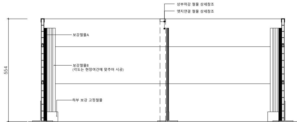
멀티엣지(W15) H550 정면도 SCALE : A1=1/6, A3=1/12
