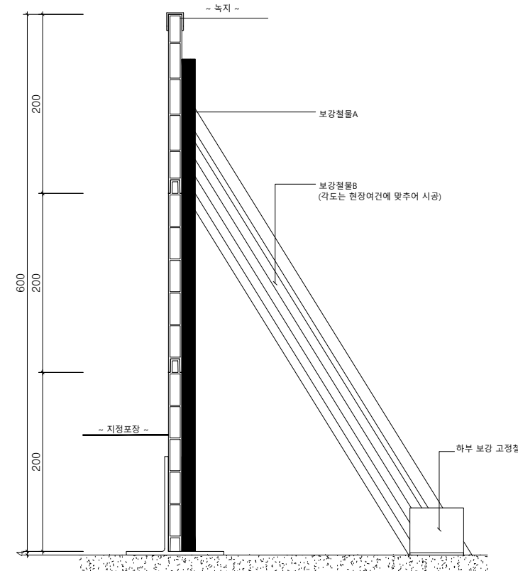
멀티엣지(W15) H600단면도
