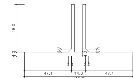
보강철물 상세도
