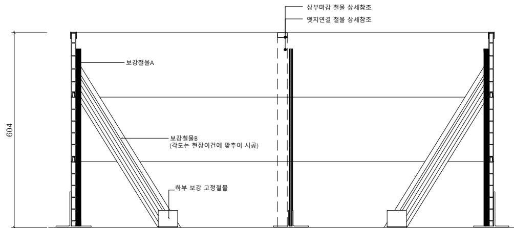
멀티엣지(W15) H600 정면도
