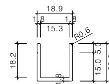
엣지상부마감철물
