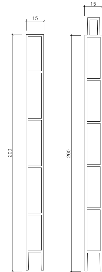
멀티엣지(W15) 알루미늄구조도(H200)
