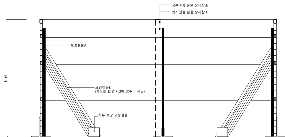
멀티엣지(W15) H650 정면도 SCALE : A1=1/6, A3=1/12
