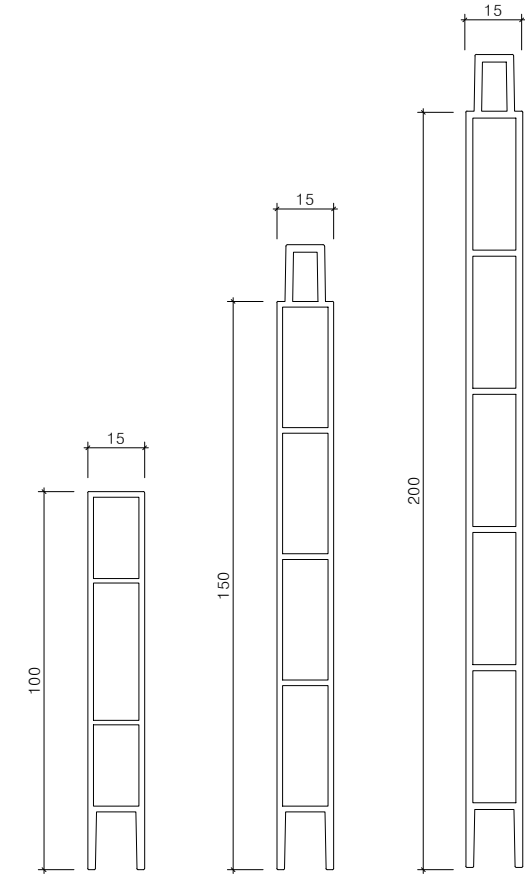
멀티엣지(W15) 알루미늄구조도(H100,150,200)도면명. SCALE : A1=1/1, A3=1/2
