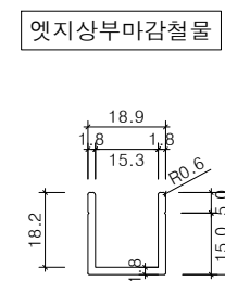
연결철물(W15) 상세도 SCALE : NONE
