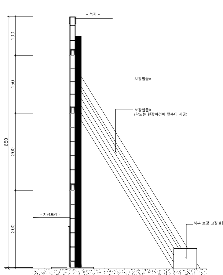
멀티엣지(W15) H650단면도 SCALE : A1=1/3, A3=1/6
