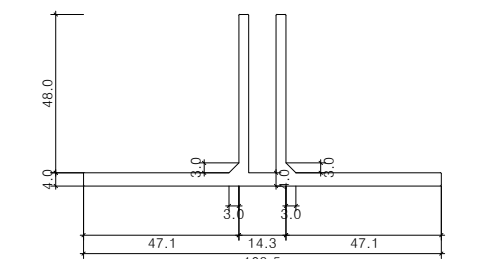
보강철물 상세도 SCALE : NONE
