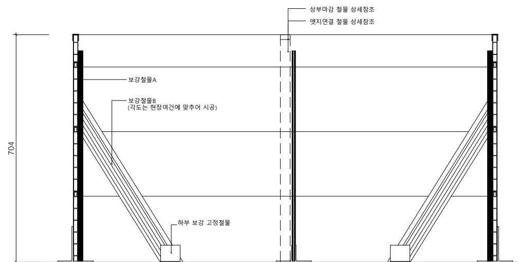
멀티엣지(W15) H700 정면도 SCALE : A1=1/6, A3=1/12
