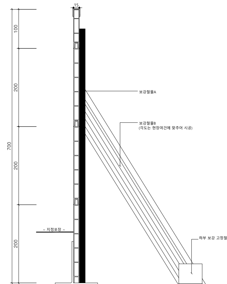
멀티엣지(W15) H700단면도 SCALE : A1=1/3, A3=1/6
