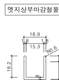
연결철물(W15) 상세도 SCALE : NONE
