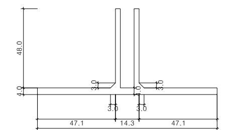
보강철물 상세도 SCALE : NONE
