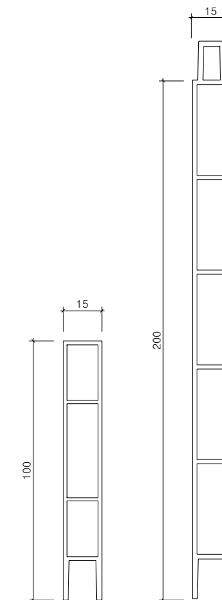
멀티엣지(W15) 알루미늄구조도(H100,200) SCALE : A1=1/1, A3=1/2
