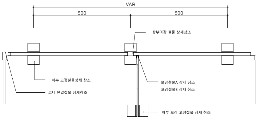
멀티엣지(W15) H700 평면도 SCALE : A1=1/6, A3=1/12
