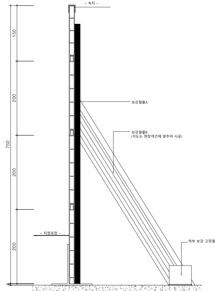
멀티엣지(W15) H750단면도 SCALE : A1=1/3, A3=1/6
