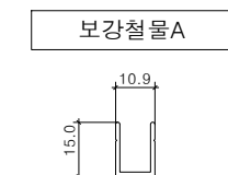
멀티엣지(W15) 알루미늄구조도(H150,200) SCALE : A1=1/1, A3=1/2
