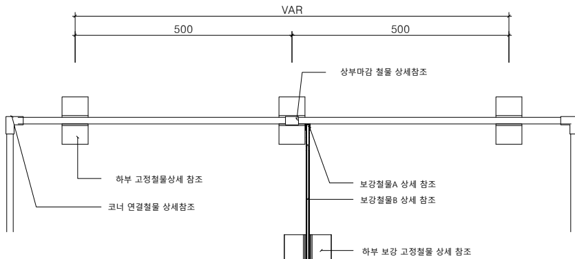
멀티엣지(W15) H750 평면도 SCALE : A1=1/6, A3=1/12
