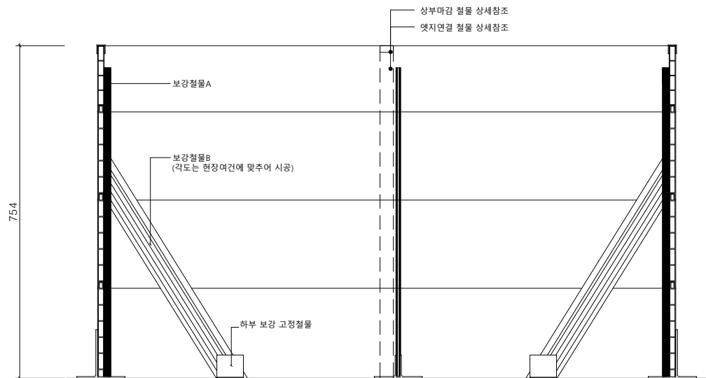
멀티엣지(W15) H750 정면도 SCALE : A1=1/6, A3=1/12
