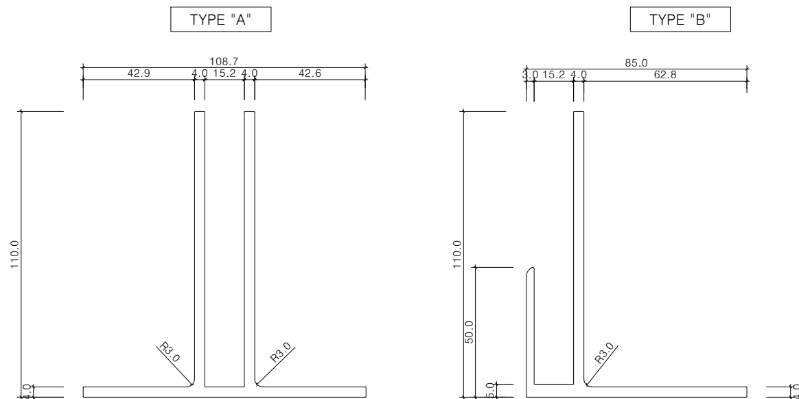
하부고정철물(W15) 상세도 SCALE : A1=1/1, A3=1/2
