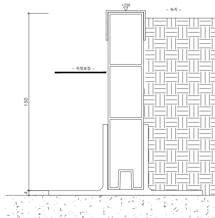
멀티엣지(W30) H150 단면도
