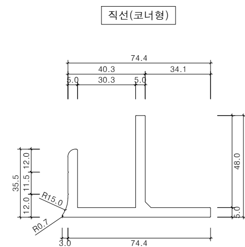
하부고정철물(W30) 상세도 SCALE : A1=1/1, A3=1/2
