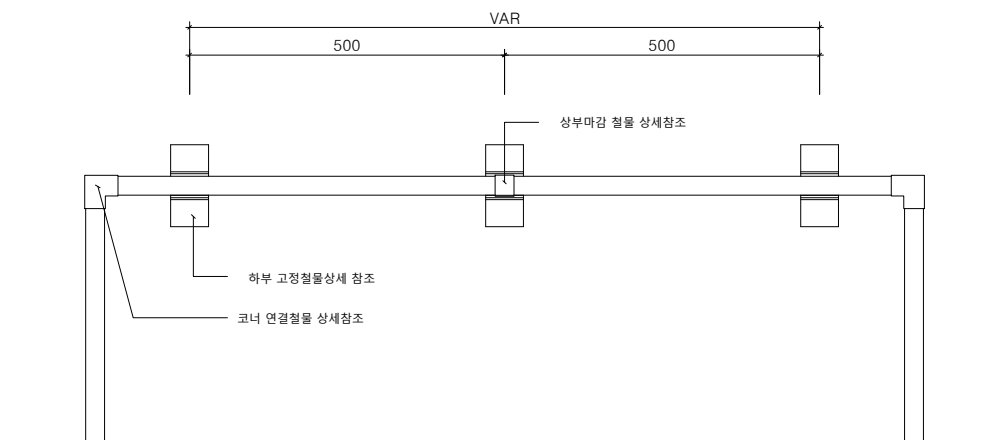
멀티엣지(W30) H150 평면도
