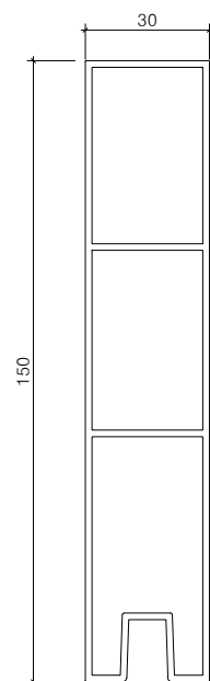
멀티엣지(W30) 알루미늄구조도(H150) SCALE : A1=1/1, A3=1/2
