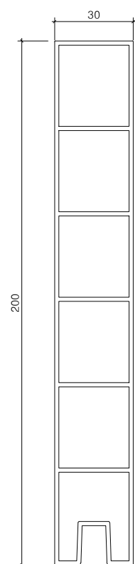
멀티엣지(W30) 알루미늄구조도(H200) SCALE : A1=1/1, A3=1/2
