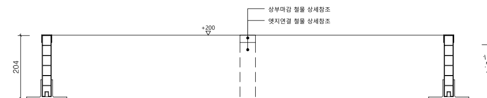
멀티엣지(W30) H200 정면도 SCALE : A1=1/6, A3=1/12
