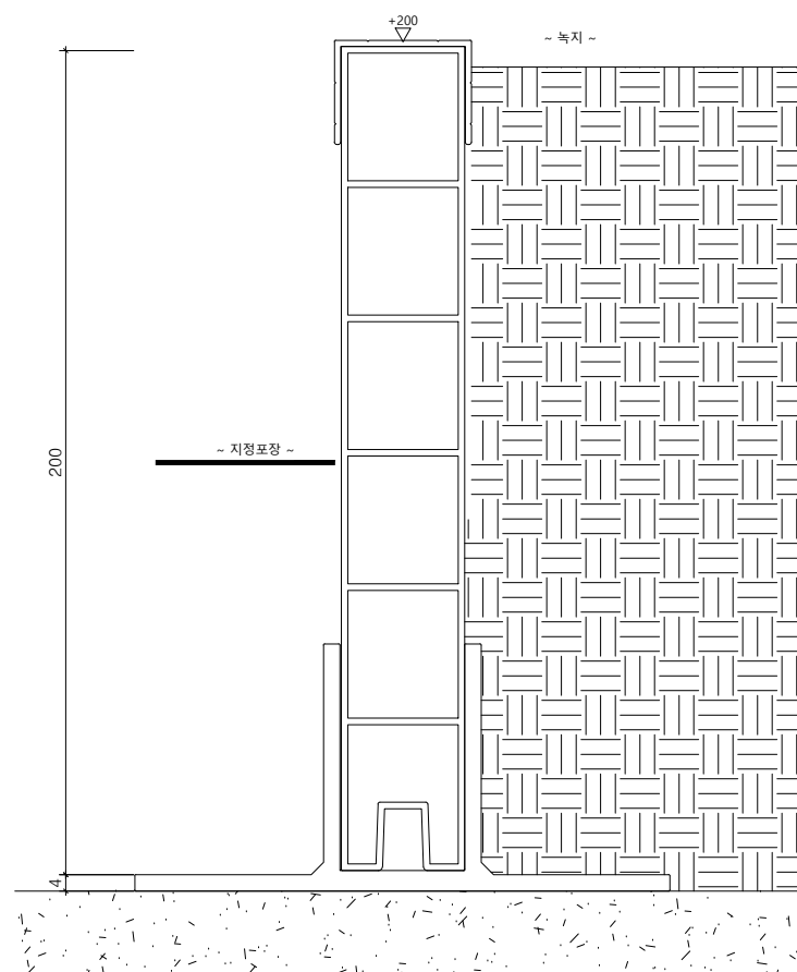
멀티엣지(W30) H200 단면도 SCALE : A1=1/1, A3=1/2
