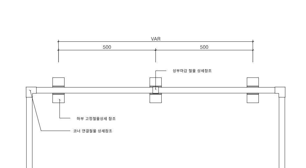
멀티엣지(W30) H200 평면도
