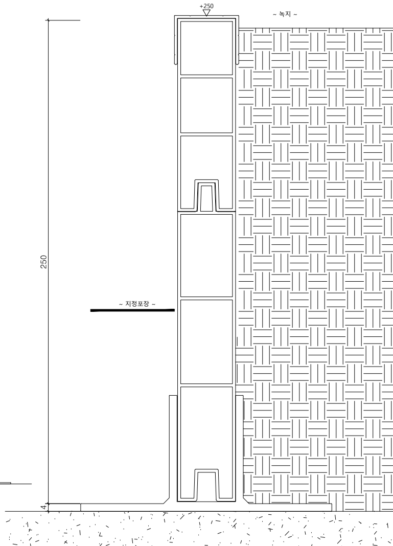
멀티엣지(W30) H250 단면도 SCALE : A1=1/1, A3=1/2
