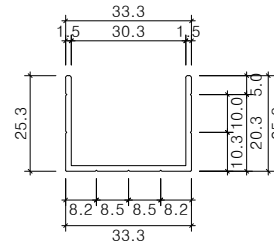
엣지상부마감철물
