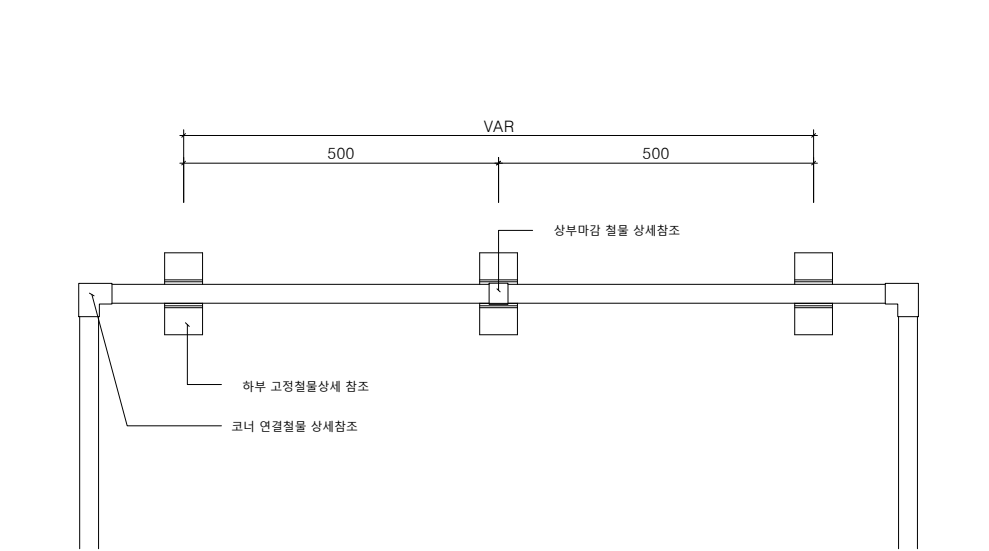
멀티엣지(W30) H250 평면도 SCALE : A1=1/6, A3=1/12
