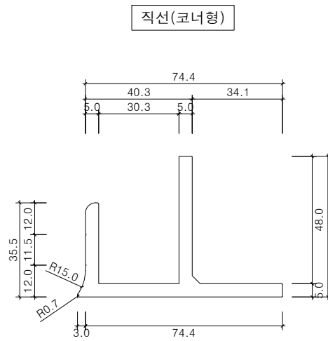
하부고정철물(W30) 상세도 SCALE : A1=1/1, A3=1/2
