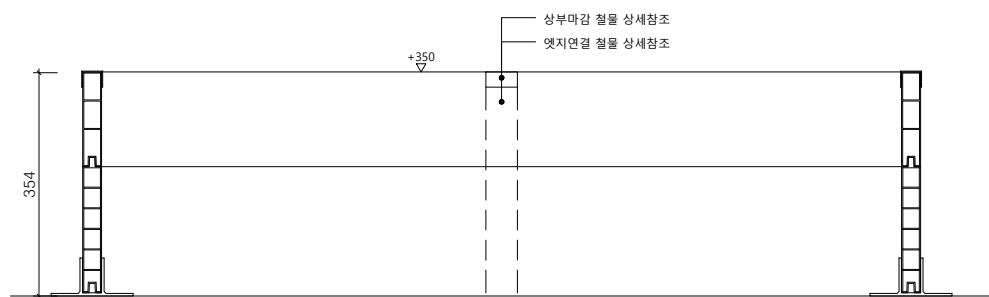
멀티엣지(W30) H350 정면도 SCALE : A1=1/6, A3=1/12
