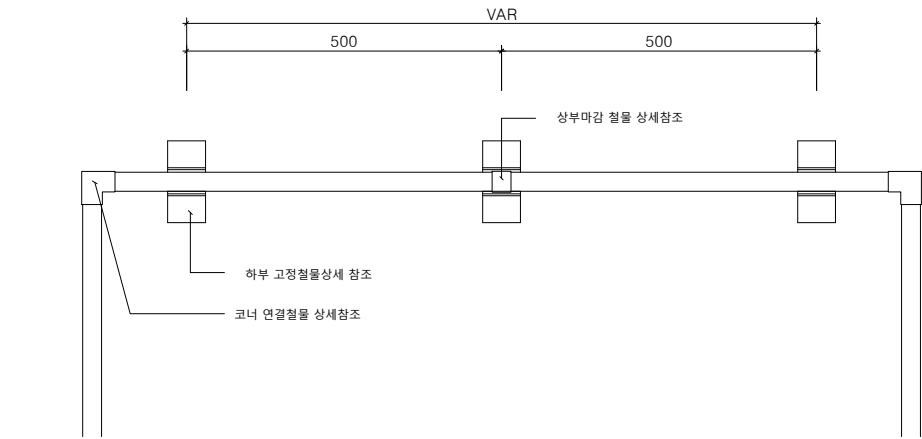
멀티엣지(W30) H350 평면도 SCALE : A1=1/6, A3=1/12
