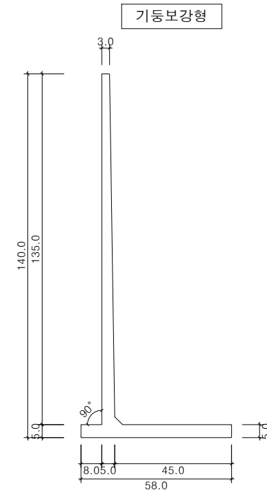
하부고정철물(W30) 상세도 SCALE : A1=1/1, A3=1/2
