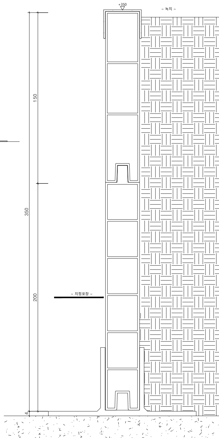
멀티엣지(W30) H350 단면도 SCALE : A1=1/1, A3=1/2
