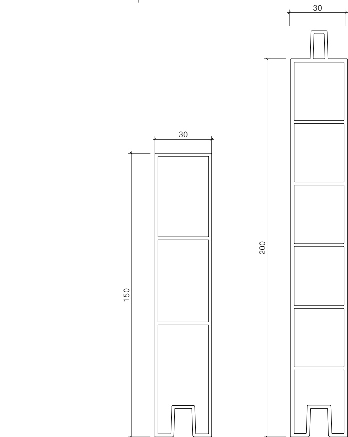
멀티엣지(W30) 알루미늄구조도(H150,200) SCALE : A1=1/1, A3=1/2
