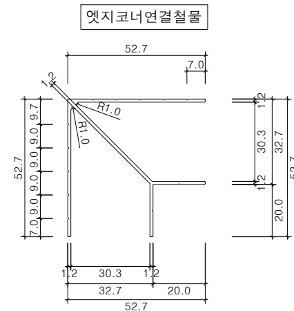
연결철물(W30) 상세도 SCALE : NONE
