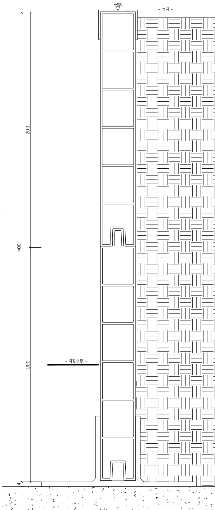
멀티엣지(W30) H400 단면도 SCALE : A1=1/1, A3=1/2
