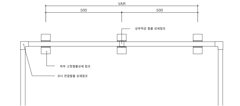
멀티엣지(W30) H400 평면도 SCALE : A1=1/6, A3=1/12
