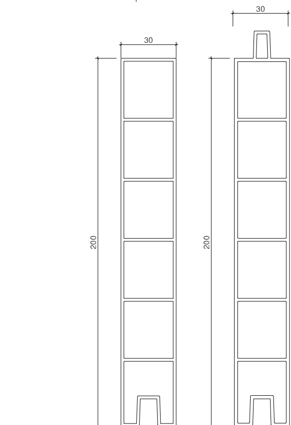
멀티엣지(W30) 알루미늄구조도(H200) SCALE : A1=1/1, A3=1/2
