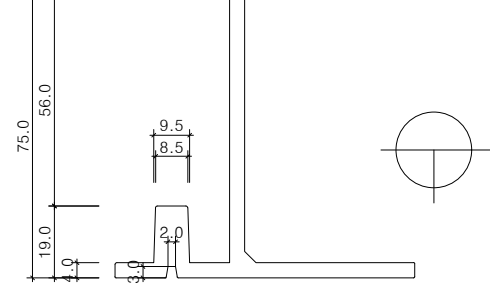
하부고정철물(W30) 상세도 SCALE : A1=1/1, A3=1/2
