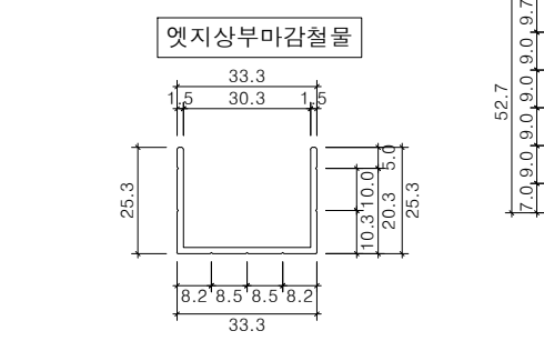
연결철물(W30) 상세도 SCALE : NONE
