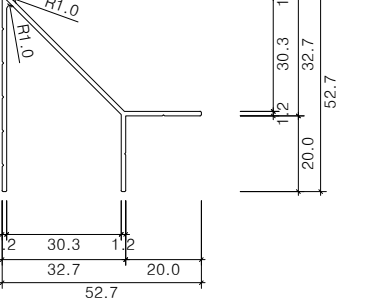
연결철물(W30) 상세도 SCALE : NONE
