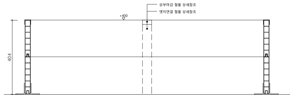
멀티엣지(W30) H400 정면도 SCALE : A1=1/6, A3=1/12
