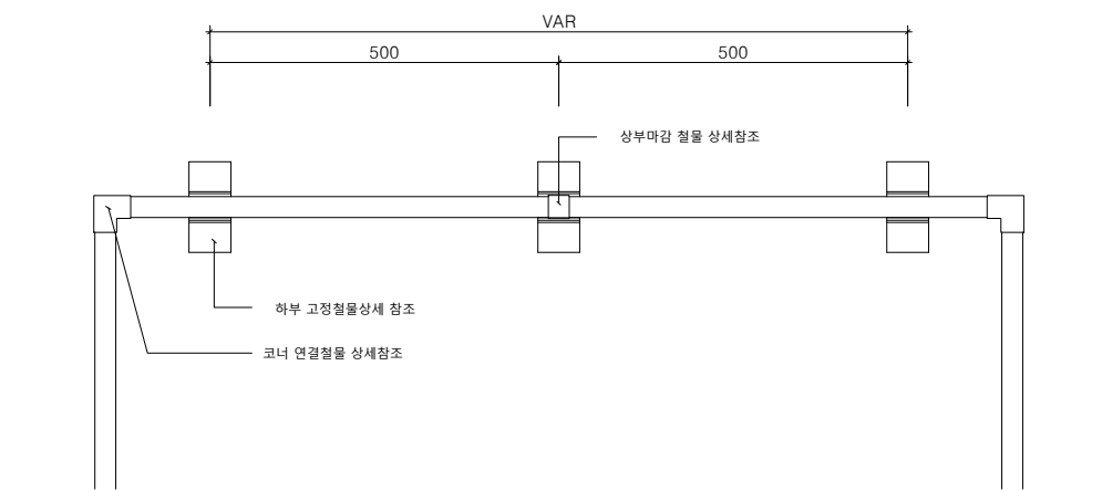
멀티엣지(W30) H450 평면도 SCALE : A1=1/6, A3=1/12
