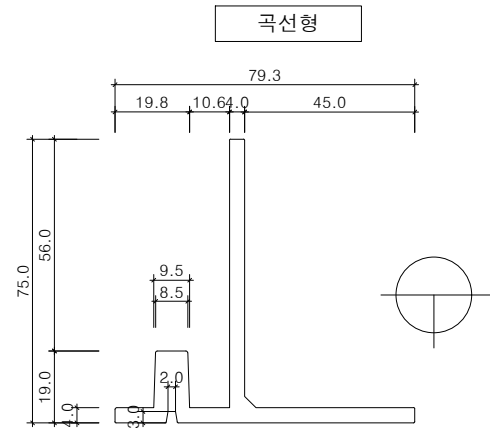
하부고정철물(W30) 상세도 SCALE : A1=1/1, A3=1/2
