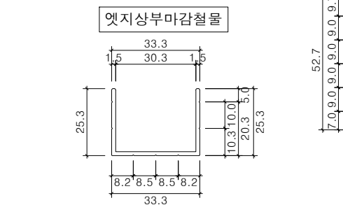
연결철물(W30) 상세도 SCALE : NONE
