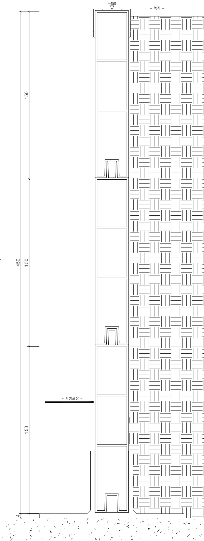
멀티엣지(W30) H450 단면도 SCALE : A1=1/1, A3=1/2
