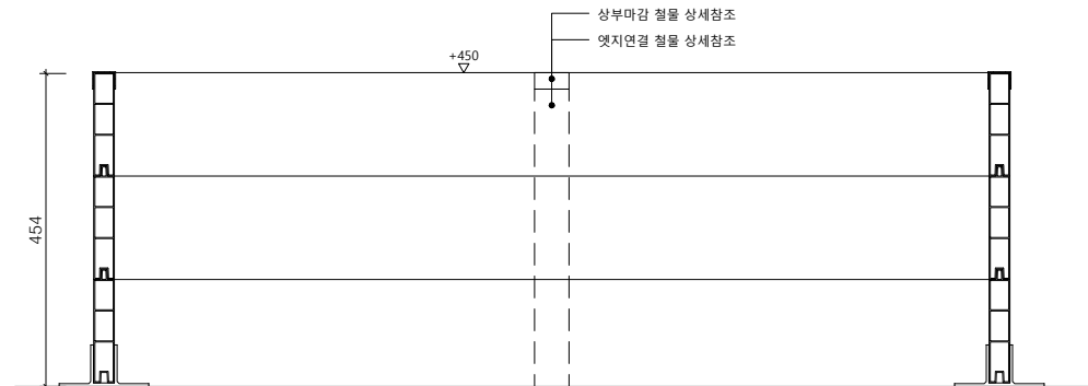
멀티엣지(W30) H450 정면도 SCALE : A1=1/6, A3=1/12
