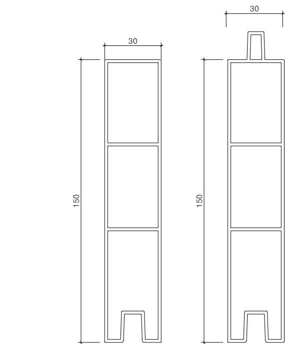
멀티엣지(W30) 알루미늄구조도(H150) SCALE : A1=1/1, A3=1/2
