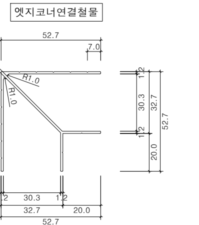
연결철물(W30) 상세도 SCALE : NONE
