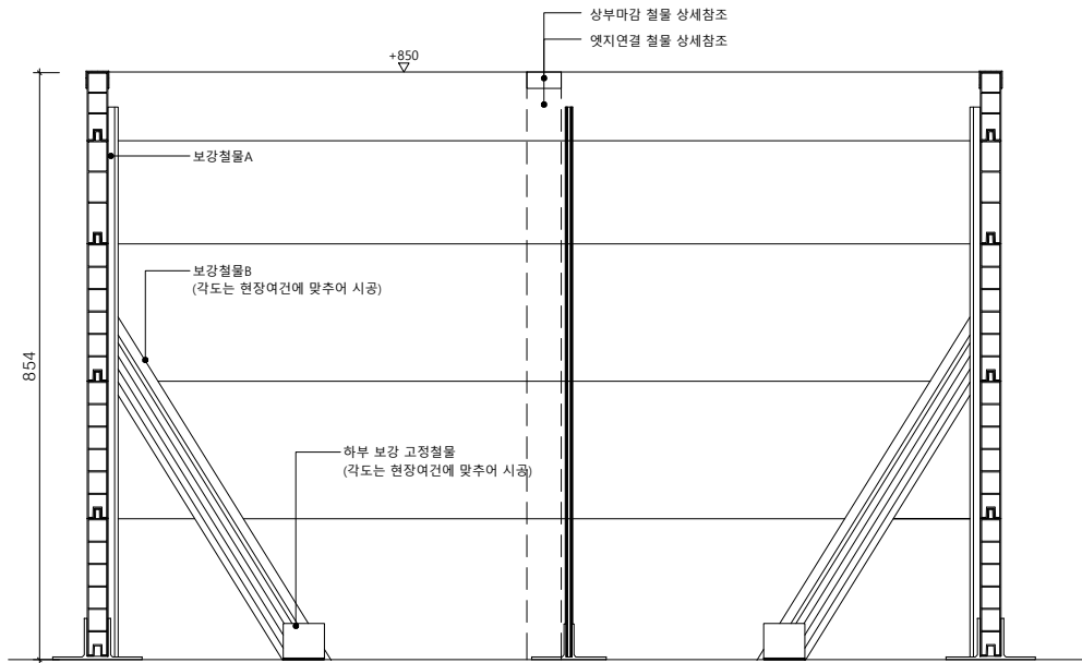
멀티엣지(W30) H850 정면도 SCALE : A1=1/6, A3=1/12
