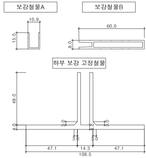
보강철물(W30) 상세도 SCALE : NONE
