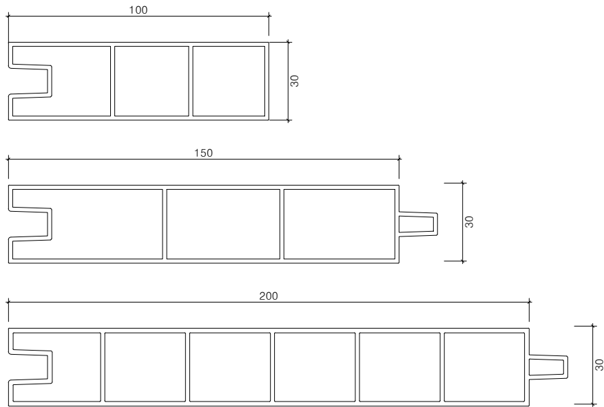
멀티엣지(W30) 알루미늄구조도(H100,150,200) SCALE : A1=1/1, A3=1/2
