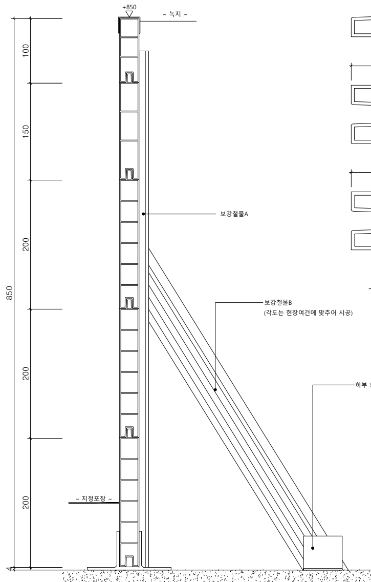
멀티엣지(W30) H850 단면도 SCALE : A1=1/3, A3=1/6
