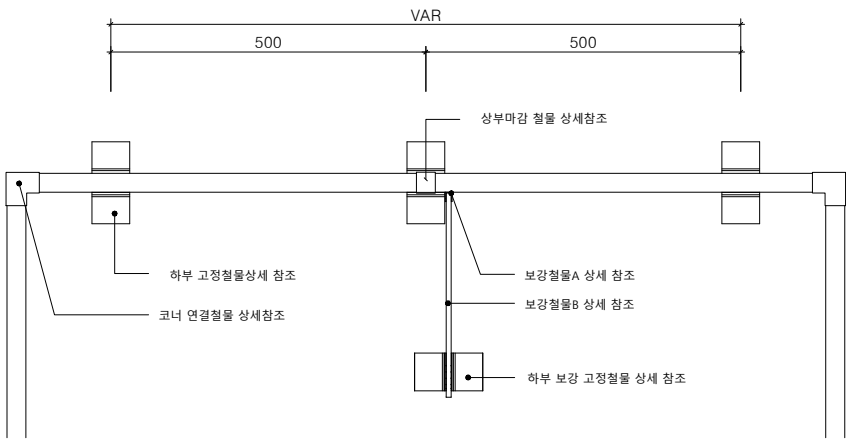
멀티엣지(W30) H850 평면도 SCALE : A1=1/6, A3=1/12
