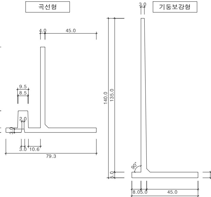
멀티엣지(W30) H850 단면도 SCALE : A1=1/3, A3=1/6
