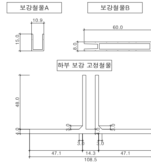
보강철물(W30) 상세도
