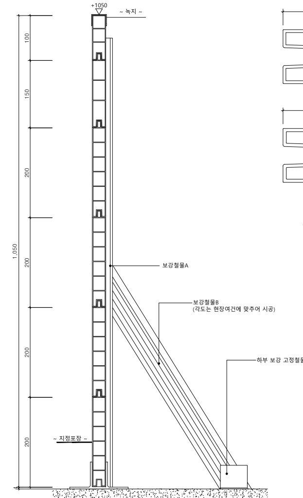
멀티엣지(W30) H1050 단면도
