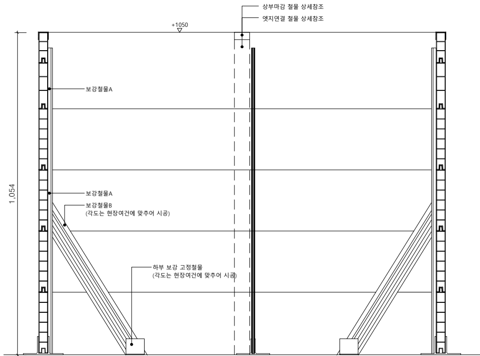
멀티엣지(W30) H1050 정면도
