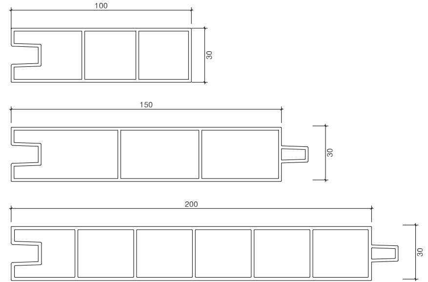
멀티엣지(W30) 알루미늄구조도(H100,150,200)
