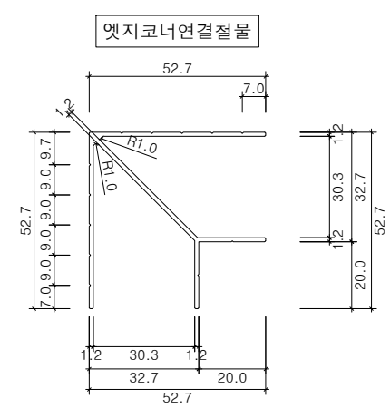
연결철물(W30) 상세도
