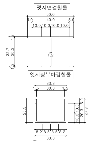
연결철물(W30) 상세도
