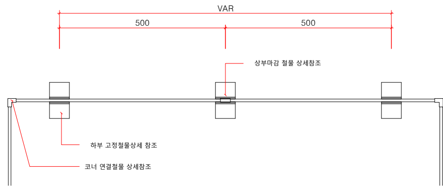
멀티엣지(W08) H60 평면도 SCALE : A1=1/6, A3=1/12
