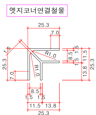
연결철물(W08) 상세도 SCALE : NONE
