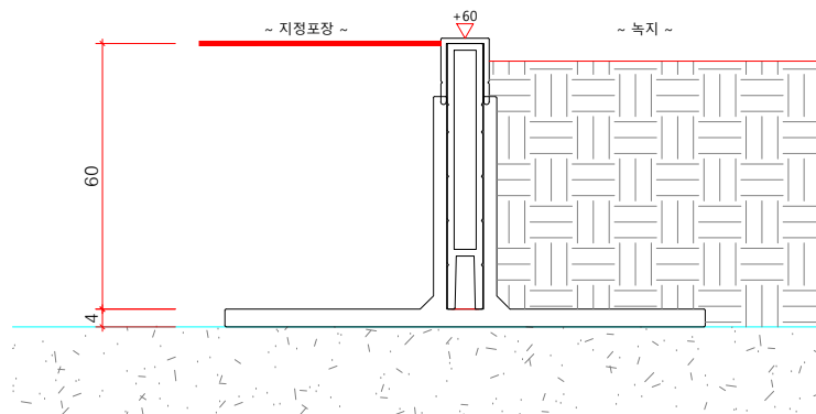
멀티엣지(W08) H80 단면도 SCALE : A1=1/1, A3=1/2
