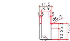
연결철물(W08) 상세도 SCALE : NONE
