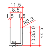
연결철물(W08) 상세도 SCALE : NONE
