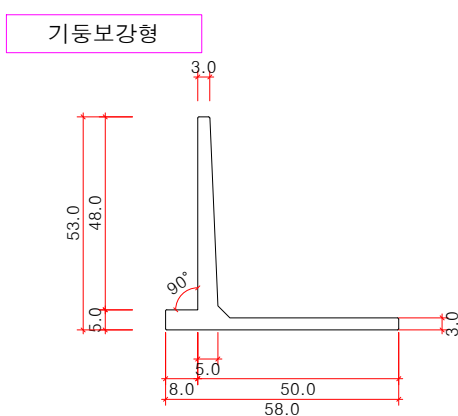
하부고정철물(W08) 상세도 SCALE : A1=1/1, A3=1/2
