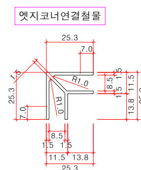
연결철물(W08) 상세도 SCALE : NONE
