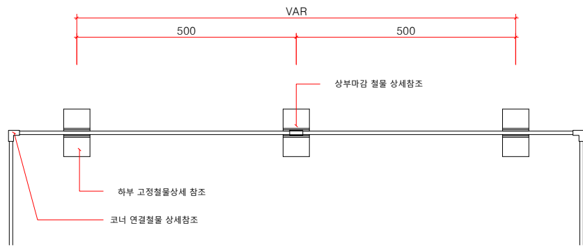
멀티엣지(W08) H80 평면도 SCALE : A1=1/6, A3=1/12
