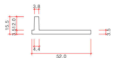
하부고정철물(W08) 상세도 SCALE : A1=1/1, A3=1/2
