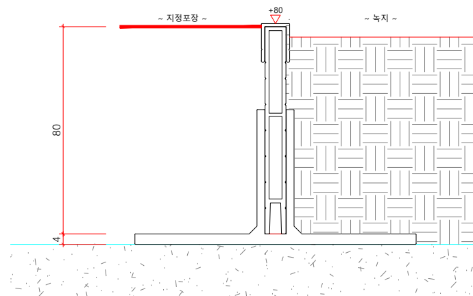
멀티엣지(W08) H80 단면도 SCALE : A1=1/1, A3=1/2
