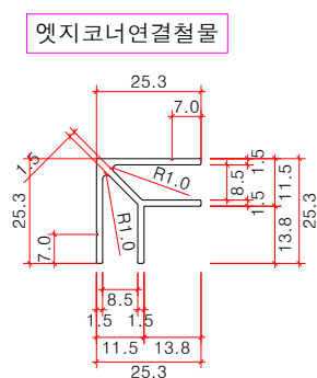
연결철물(W08) 상세도 SCALE : NONE
