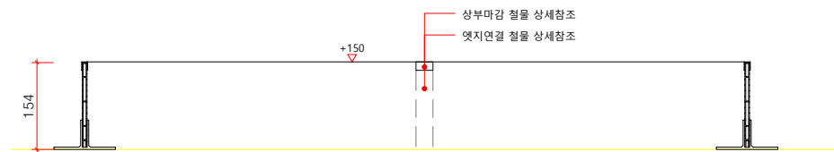
멀티엣지(W08) H150 정면도 SCALE : A1=1/6, A3=1/12
