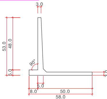
하부고정철물(W08) 상세도 SCALE : A1=1/1, A3=1/2
