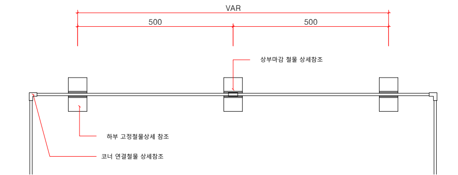
멀티엣지(W08) H150 평면도 SCALE : A1=1/6, A3=1/12
