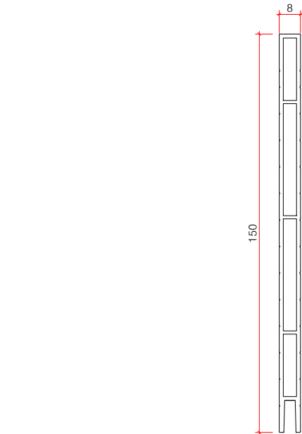
멀티엣지(W08) 알루미늄구조도(H150) SCALE : A1=1/1, A3=1/2
