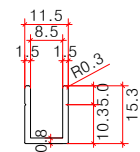
엣지상부마감철물
