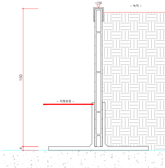
멀티엣지(W08) H150 단면도 SCALE : A1=1/1, A3=1/2
