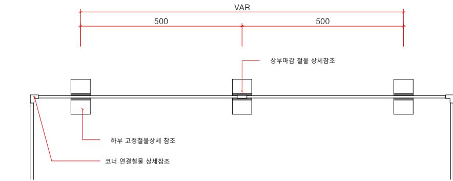
멀티엣지(W08) H200 평면도 SCALE : A1=1/6, A3=1/12
