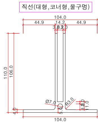
하부고정철물(W08) 상세도 SCALE : A1=1/1.5, A3=1/3
