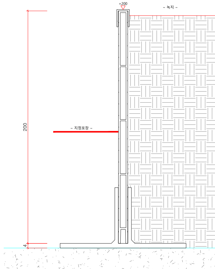
멀티엣지(W08) H200 단면도 SCALE : A1=1/1, A3=1/2
