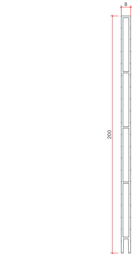
멀티엣지(W08) 알루미늄구조도(H200) SCALE : A1=1/1, A3=1/2
