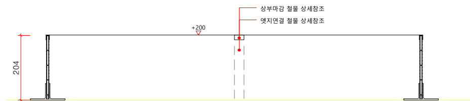
멀티엣지(W08) H200 정면도 SCALE : A1=1/6, A3=1/12
