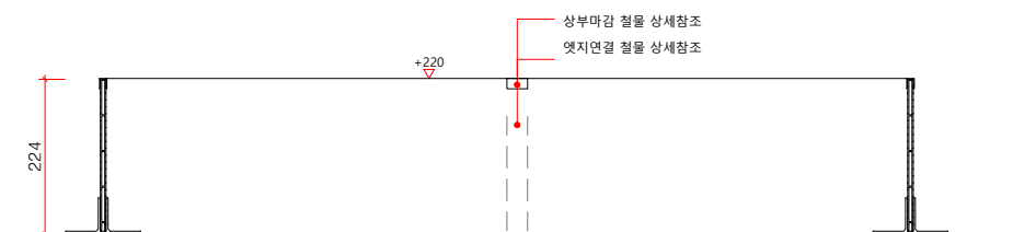
멀티엣지(W08) H220 정면도
