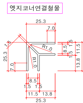
연결철물(W08) 상세도 SCALE : NONE
