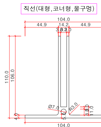
하부고정철물(W08) 상세도 SCALE : A1=1/1.5, A3=1/3
