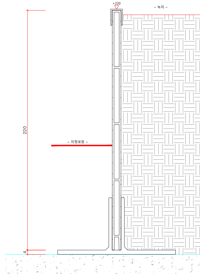
멀티엣지(W08) H220 단면도 SCALE : A1=1/1, A3=1/2
