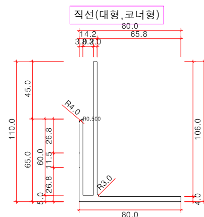
하부고정철물(W08) 상세도 SCALE : A1=1/1.5, A3=1/3
