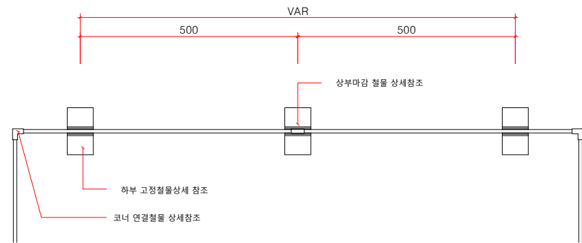
멀티엣지(W08) H220 평면도 SCALE : A1=1/6, A3=1/12
