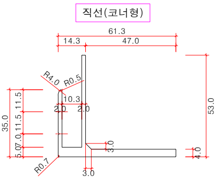
하부고정철물(W10) 상세도 SCALE : A1=1/1, A3=1/2
