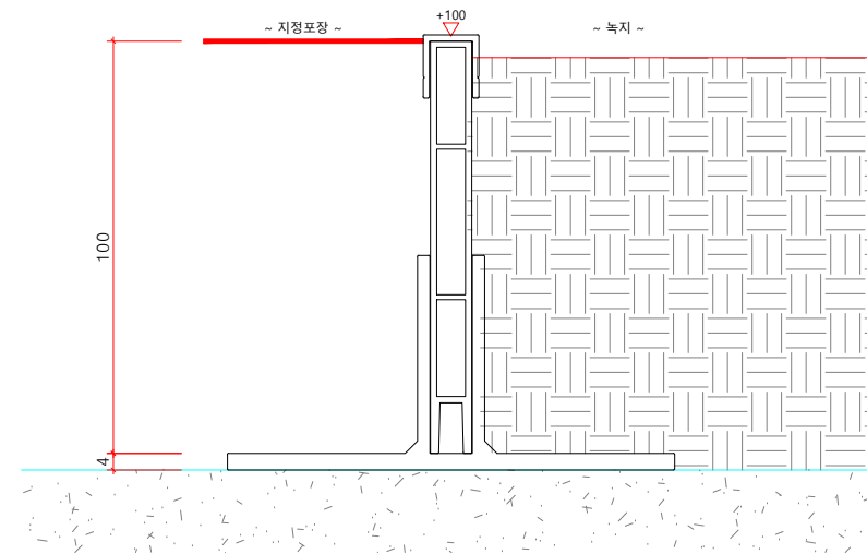
멀티엣지(W10) H100 단면도 SCALE : A1=1/1, A3=1/2
