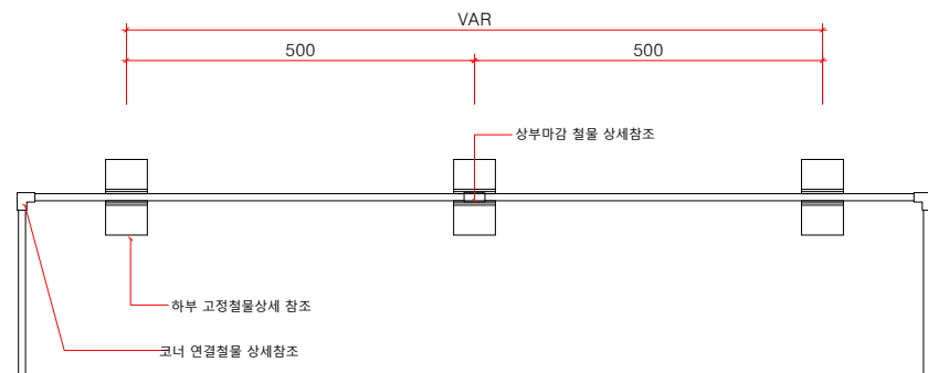
멀티엣지(W10) H150 평면도 SCALE : A1=1/6, A3=1/12
