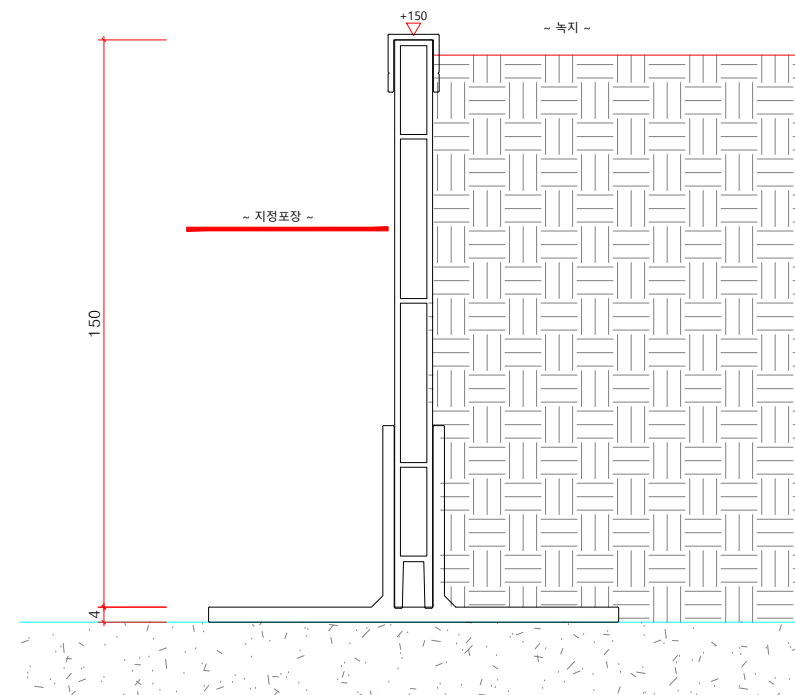
멀티엣지(W10) H150 단면도 SCALE : A1=1/1, A3=1/2
