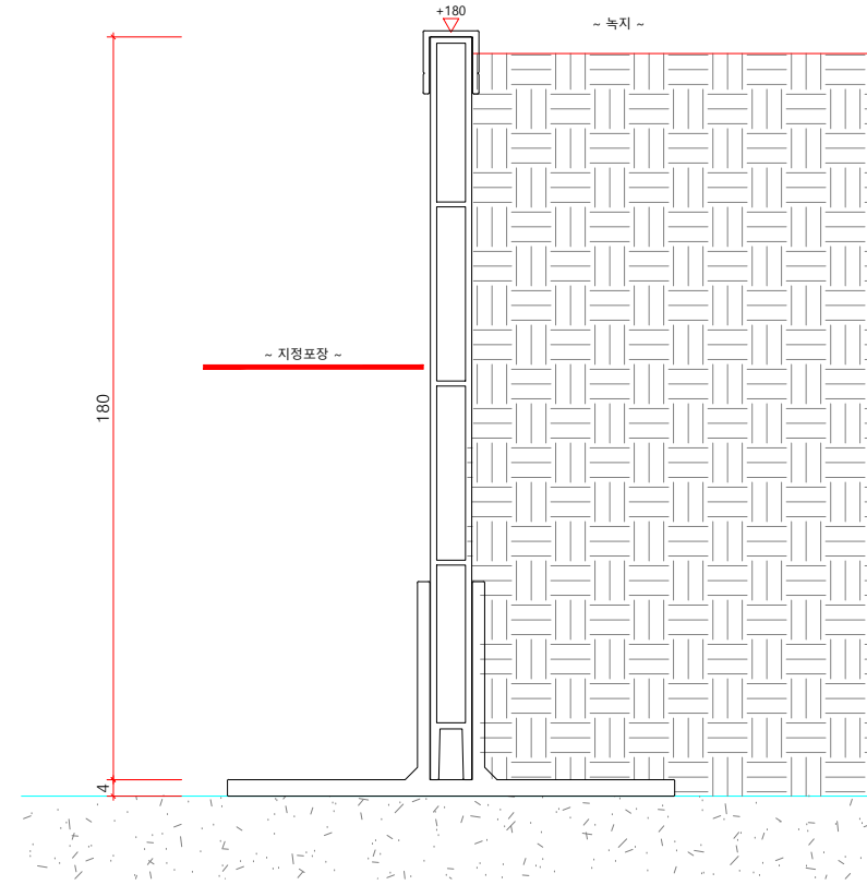
멀티엣지(W10) H180 단면도 SCALE : A1=1/1, A3=1/2
