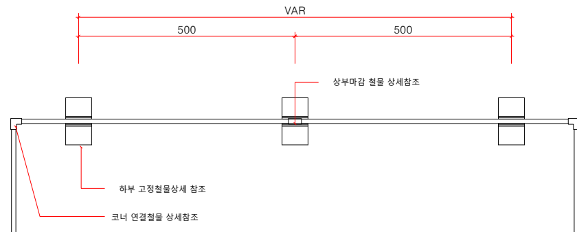
멀티엣지(W10) H180 평면도 SCALE : A1=1/6, A3=1/12
