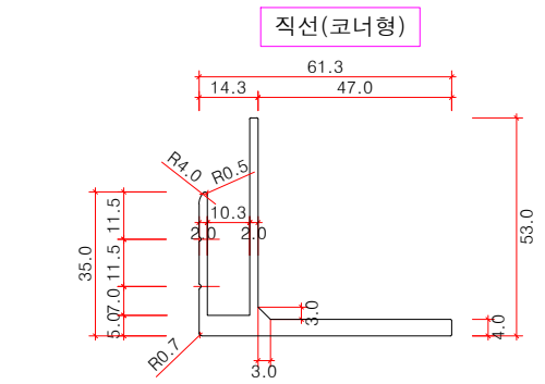
하부고정철물(W10) 상세도 SCALE : A1=1/1, A3=1/2
