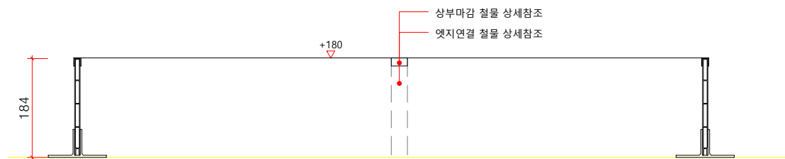
멀티엣지(W10) H180 정면도 SCALE : A1=1/6, A3=1/12
