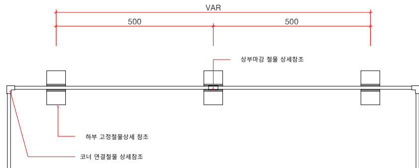
멀티엣지(W10) H250 평면도 SCALE : A1=1/6, A3=1/12
