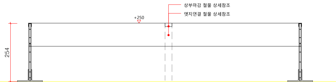
멀티엣지(W10) H250 정면도 SCALE : A1=1/6, A3=1/12
