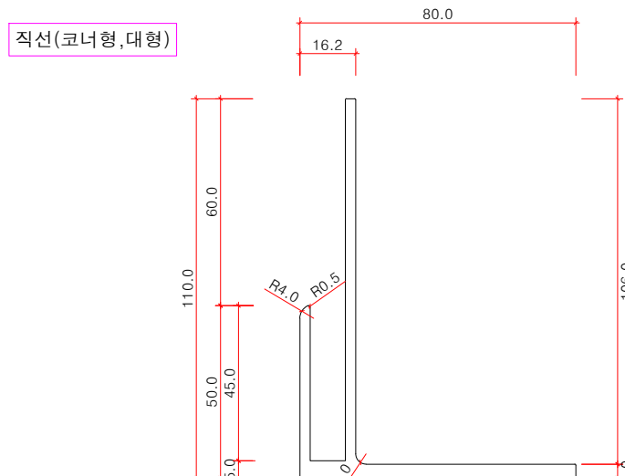
하부고정철물(W10) 상세도 SCALE : A1=1/1, A3=1/2
