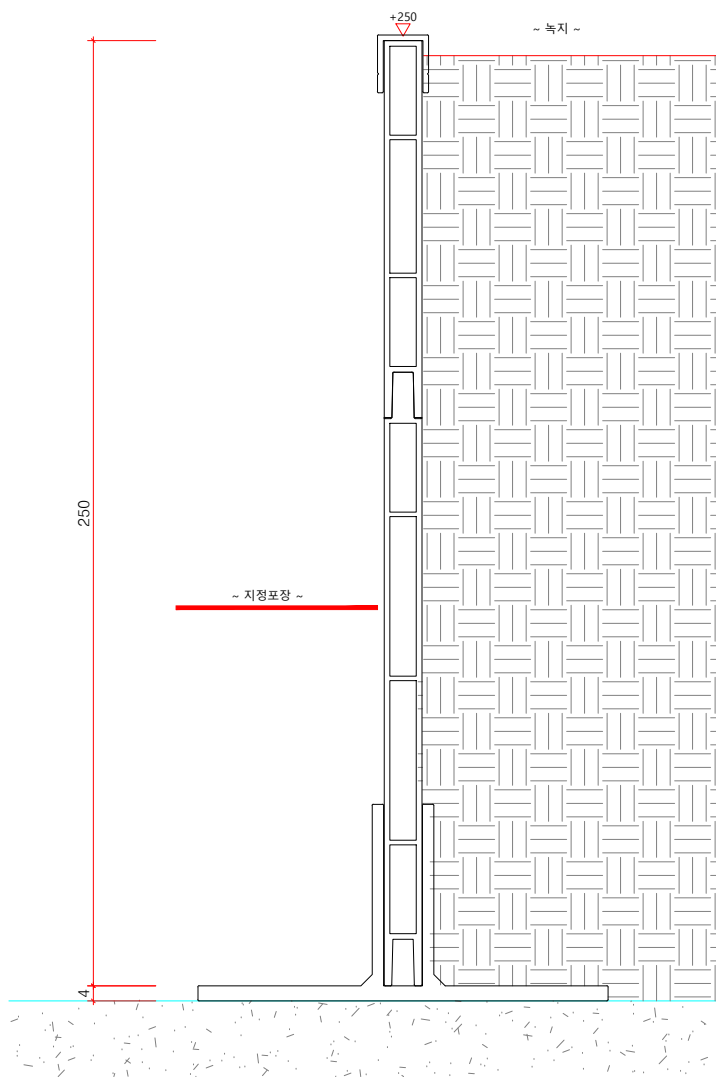
멀티엣지(W10) H250 단면도 SCALE : A1=1/1, A3=1/2
