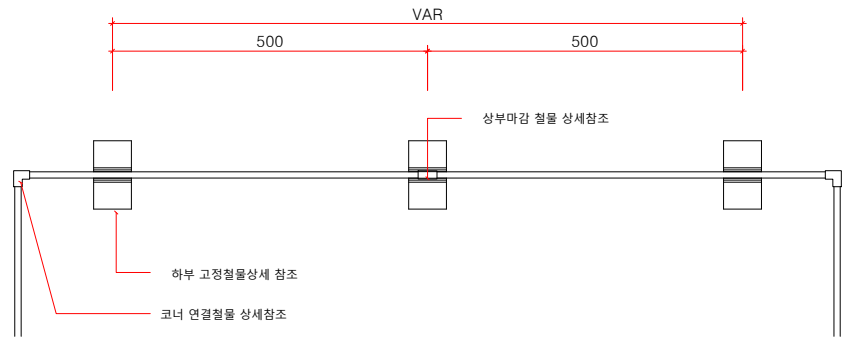
멀티엣지(W10) H300 평면도 SCALE : A1=1/6, A3=1/12
