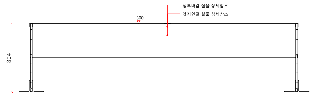
멀티엣지(W10) H300 정면도 SCALE : A1=1/6, A3=1/12
