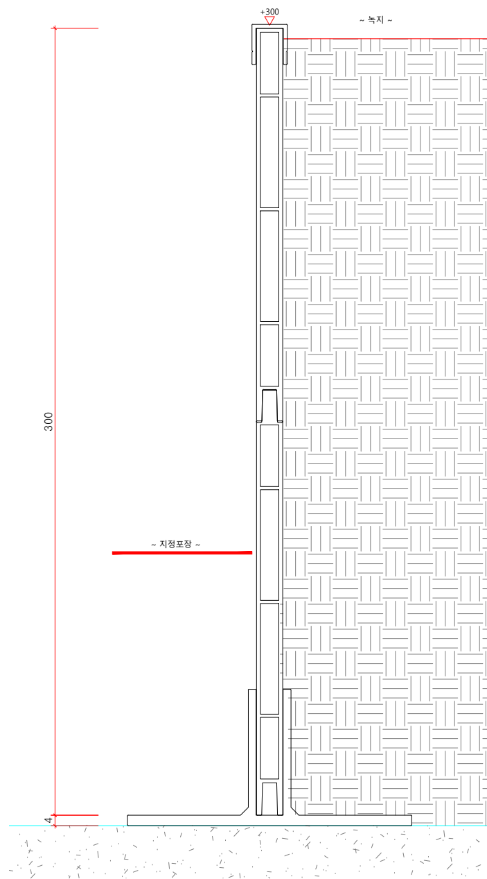
멀티엣지(W10) H300 단면도 SCALE : A1=1/1, A3=1/2
