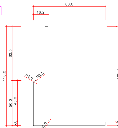
하부고정철물(W10) 상세도 SCALE : A1=1/1, A3=1/2
